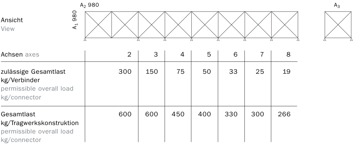
Statisches System: Beispiel 4 (A 1 980/ A 2 980 / A 3 )
