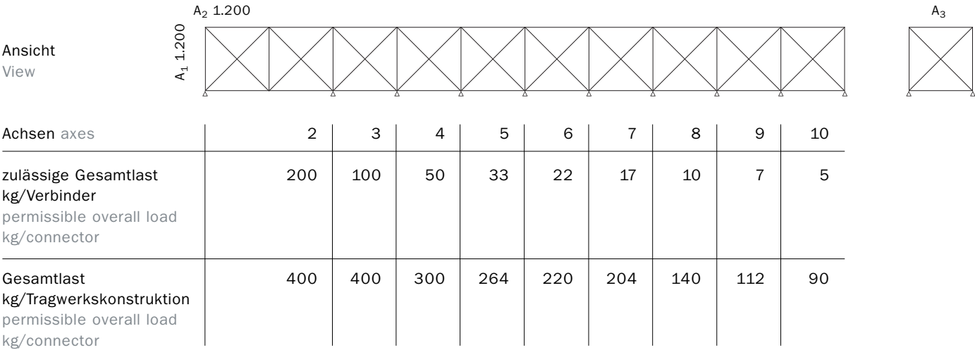
Statisches System: Beispiel 2 (A 1 1.200/ A 2 1.200 / A 3 )
